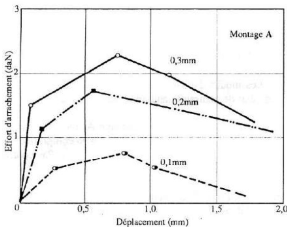
Figure 4 : Courbe effort d'arrachement-déplacement (Montage A).
