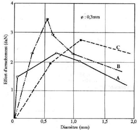
Figure 16 : Influence du mode d'essai sur l'allure de la courbe effort d'arrachement-déplacement dans le cas du diamètre de 0,3mm.
