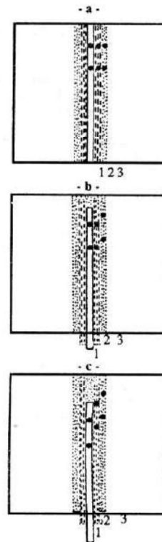
Figure 9 : Schéma d'explication physique du phénomène de fracture de la matrice pendant la phase de retrait.
