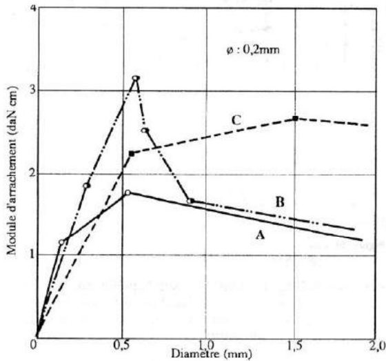
Figure 15 : Influence du mode d'essai sur l'allure de la courbe effort d'arrachement-déplacement dans le cas du diamètre de 0,2mm.
