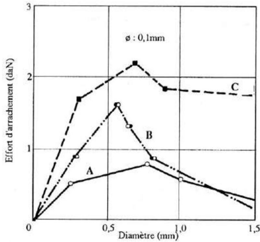
Figure 14 : Influence du mode d'essai sur l'allure de la courbe effort d'arrachement-déplacement dans le cas du diamètre de 0,1mm.
