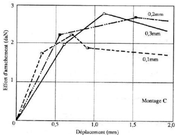
Figure 8 : Courbe effort d'arrachement-déplacement (Montage C).
