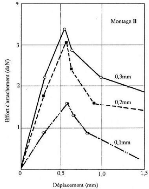
Figure 5 : Courbe effort d'arrachement-déplacement (Montage B).
